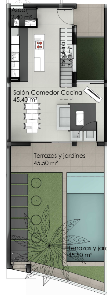
Planta Baja
