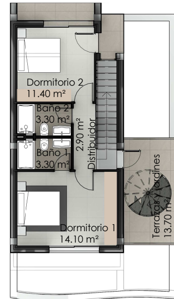
Planta Primera
