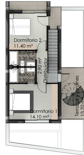
Planta Primera
