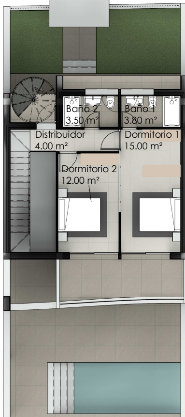
Planta Primera
