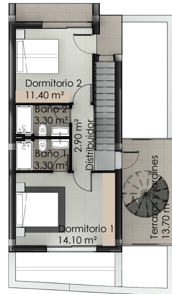
Planta Primera
