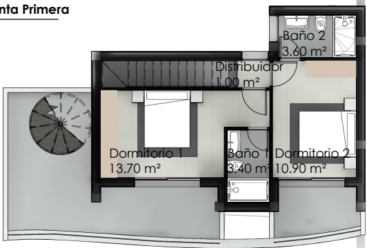
Planta Primera
